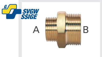
Nipplo ridotti M/M in ottone con doppia filettatura maschio ISO 228 G a battuta piana (A-B)
