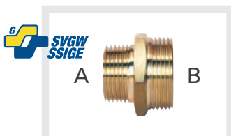
Nipplo ridotti M/M in ottone con filettatura maschio ISO 228 G a battuta piana (B) e filettatura maschio conica EN 10226 R (A)
