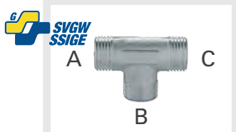
Raccordi TEE M/M/M in ottone nichelato con filettatura maschio ISO 228 G a battuta piana (A-B-C)
