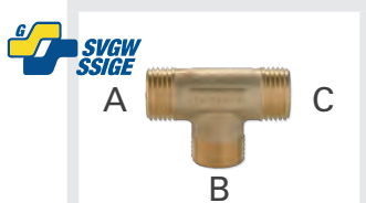
Raccordi TEE M/M/M in ottone con filettatura maschio ISO 228 G a battuta piana (A-B-C)
